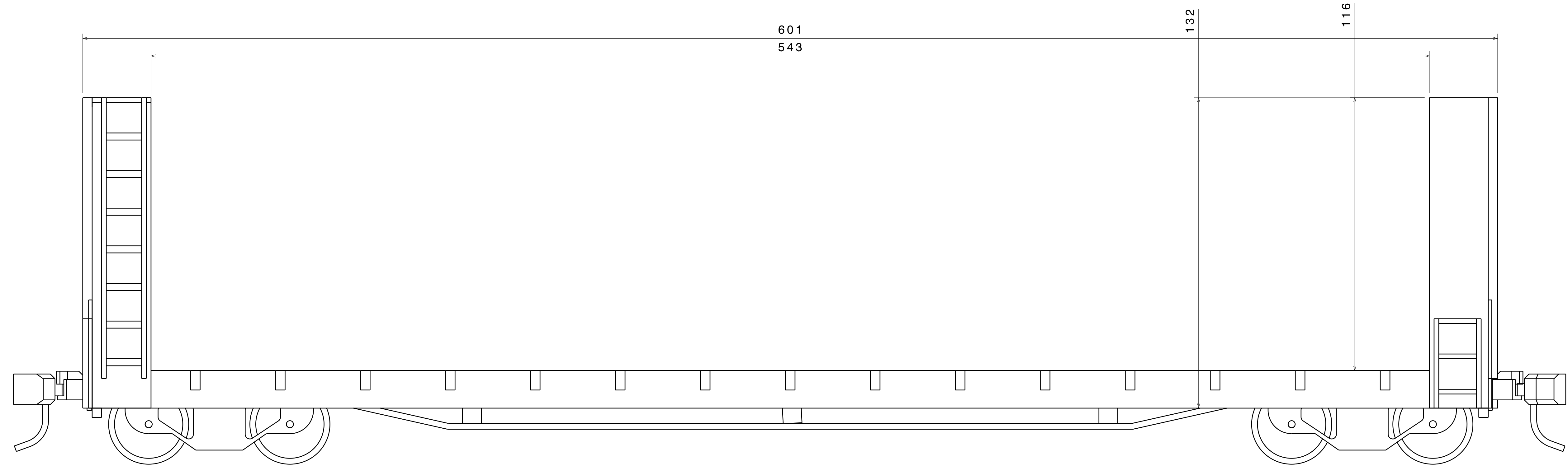
Front view Scale: 1:1
